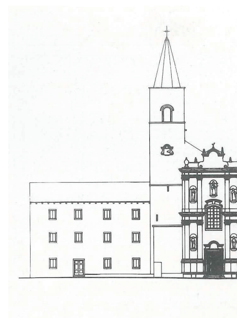
Nacrt pročelja crkve i samostana te uzdužni presjek crkve Nacrt pročelja crkve i samostana te vzdolžni presek crkve
