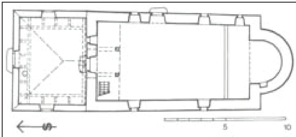
Kapela, tlocrt Tloris kapele
