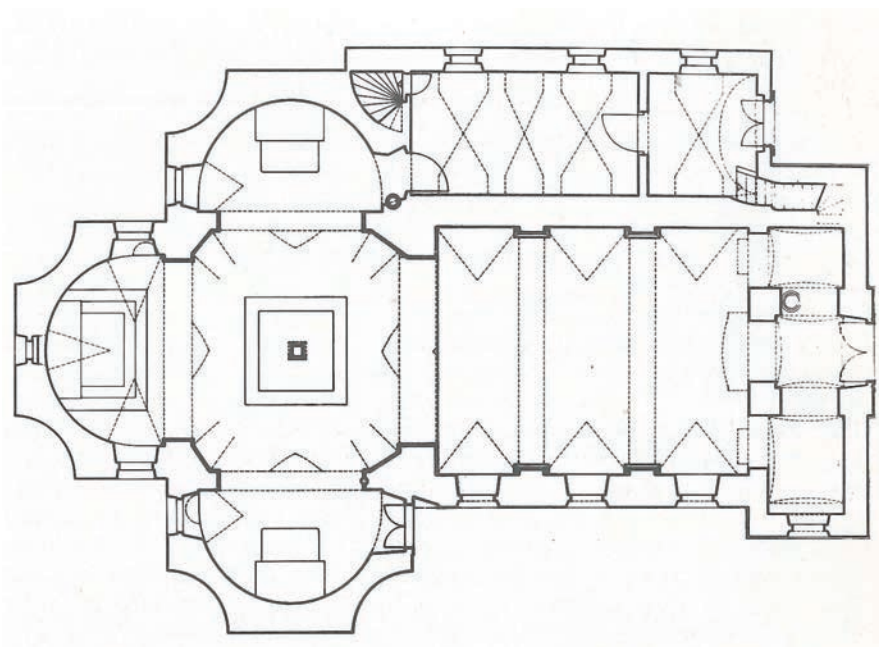
Kapela, tlocrt Tloris kapele
