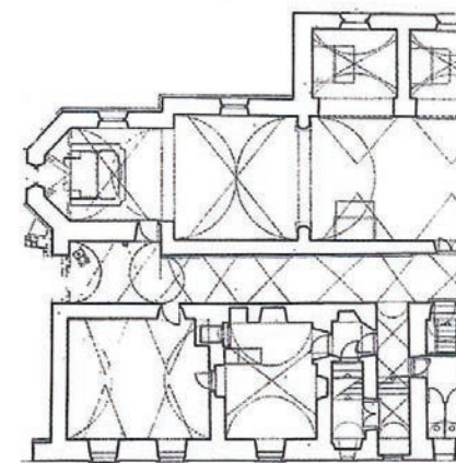
Tlocrt samostana i crkve Tloris samostana in cerkve
