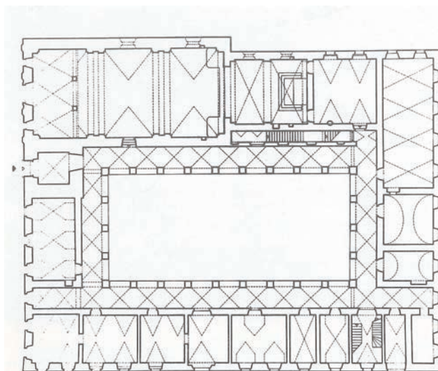
Tlocrt samostana Tloris samostana
