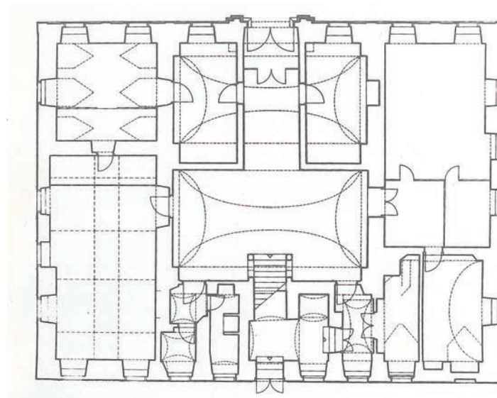
Pavlinski marof, tlocrt prizemlja kurije Pavlinška pristava, tloris pritlička dvorca
