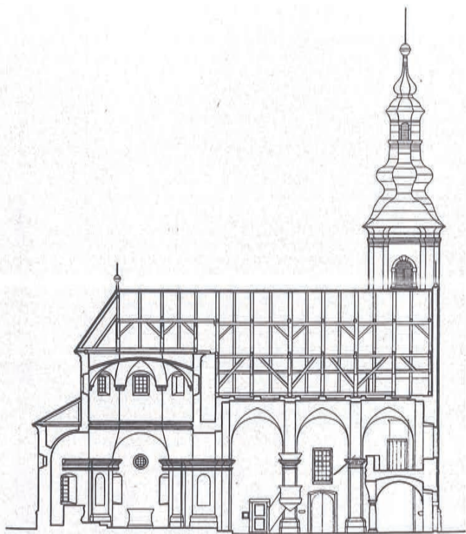
Uzdužni presjek crkve Vzdolžni prerez cerkve
