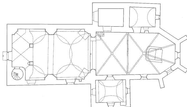
Tlocrt crkve Tloris crkve
